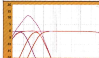
Sinnvolle Auslegung der Filter. Auch Kickbässe lassen sich per Bandpass ansteuern
